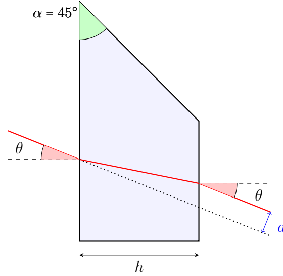
Figura 3: Schema della deviazione di un raggio incidente in un prisma a base trapezoidale
